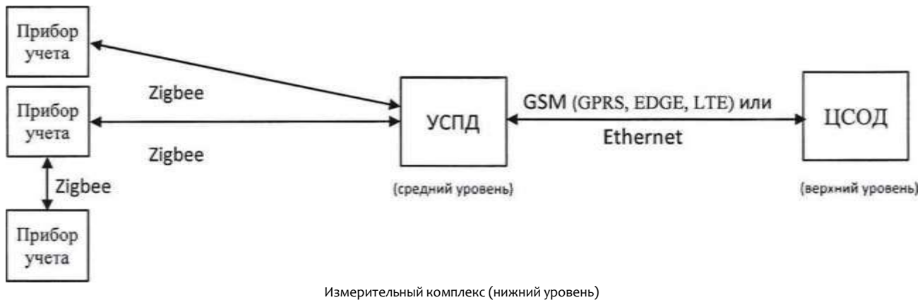
Измерительный комплекс (нижний уровень)
